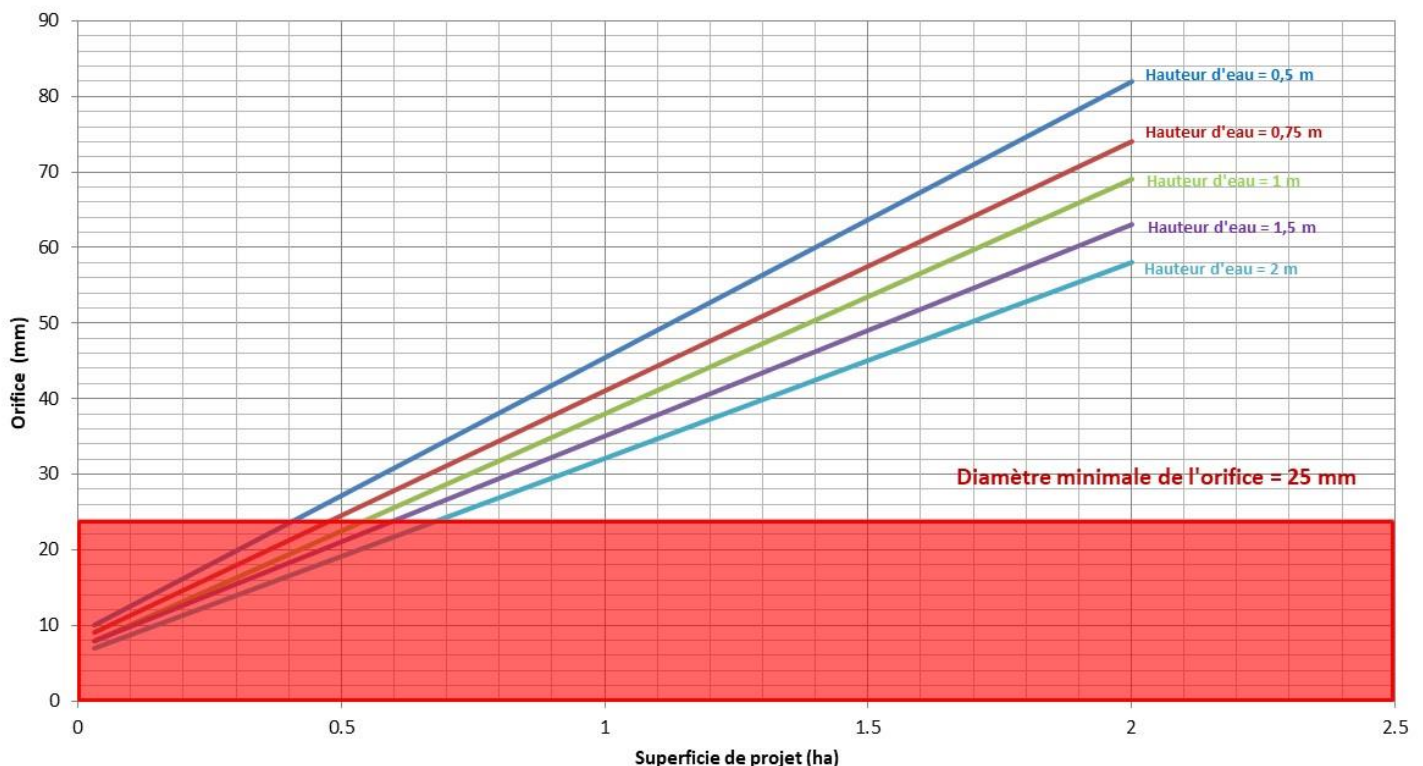
Détermination de l'orifice de l'ouvrage de rétention
